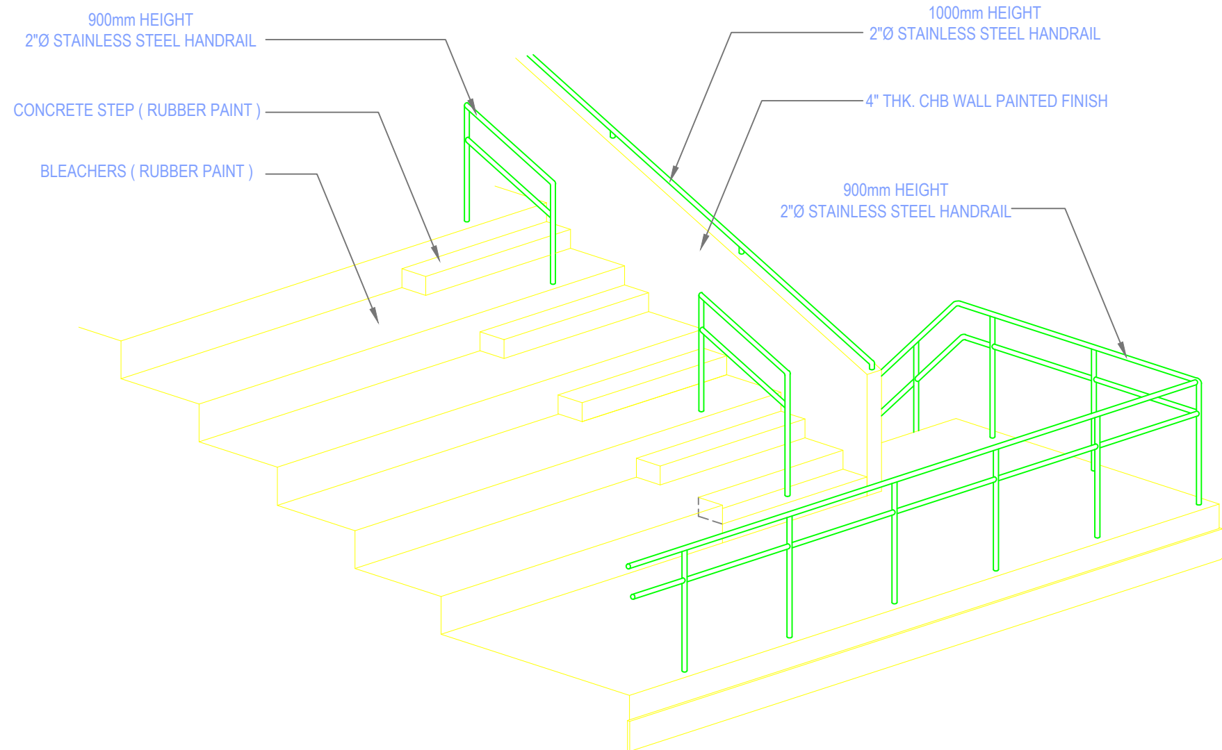
ISOMETRIC VIEW OF BLEACHERS N. T. S.
