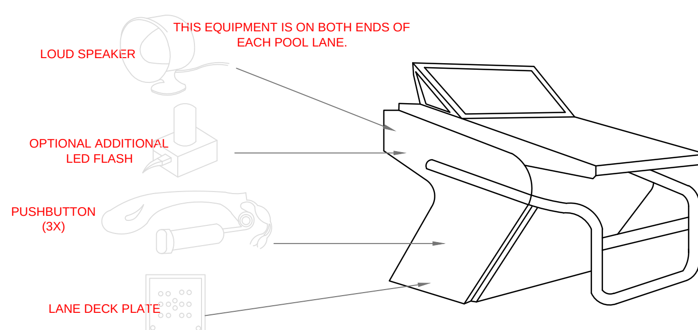
DETAIL OF STARTING BLOCK N. T. S.
