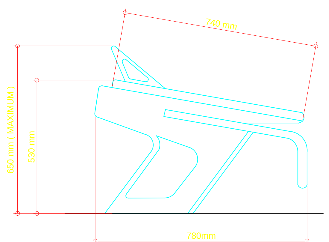
DETAIL OF STARTING BLOCK N. T. S.
