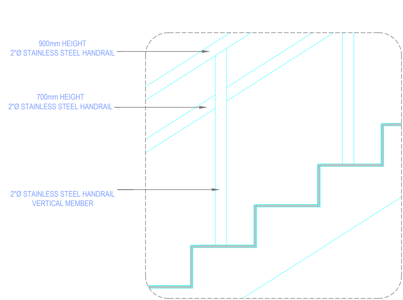
DETAIL OF RAILING N. T. S.
